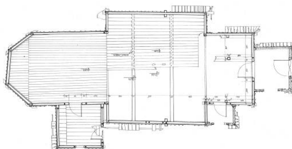
Ryc. 4a. Cerkiew w Mięksiz Starym, gm. Laszki – rysunki inwentaryzacyjne wykonane przez studentów architektury Politechniki Krakowskiej pod kierunkiem autora: rzut parteru /J.Sowa/.
