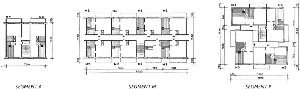
Fig. 5. Examples of ready-made plans. Source: [7] Ryc. 5. Przykładowe schematy gotowych rzutów. Źródło: [7]
