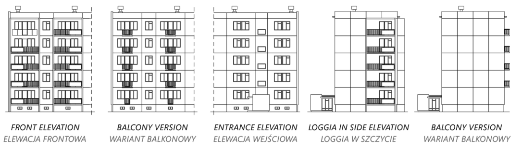
Fig. 3. Example elevations of a five-story building (right segment "A"). Source: [6] Ryc. 3. Przykładowe elewacje budynku 5-kondygnacyjnego (segment skrajny prawy „A”). Źródło: [6]
